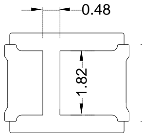
Fig.1-3 Bottom view 背面视图 Fig.1-4 Polarity 极性
