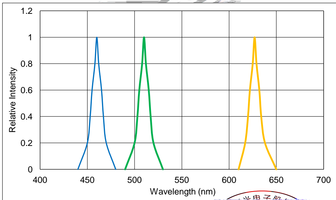
Fig.1-13 Relative Intensity Vs Wavelength (Ta=25°C) 相对光强与波长关系曲线 (Ta=25°C)
